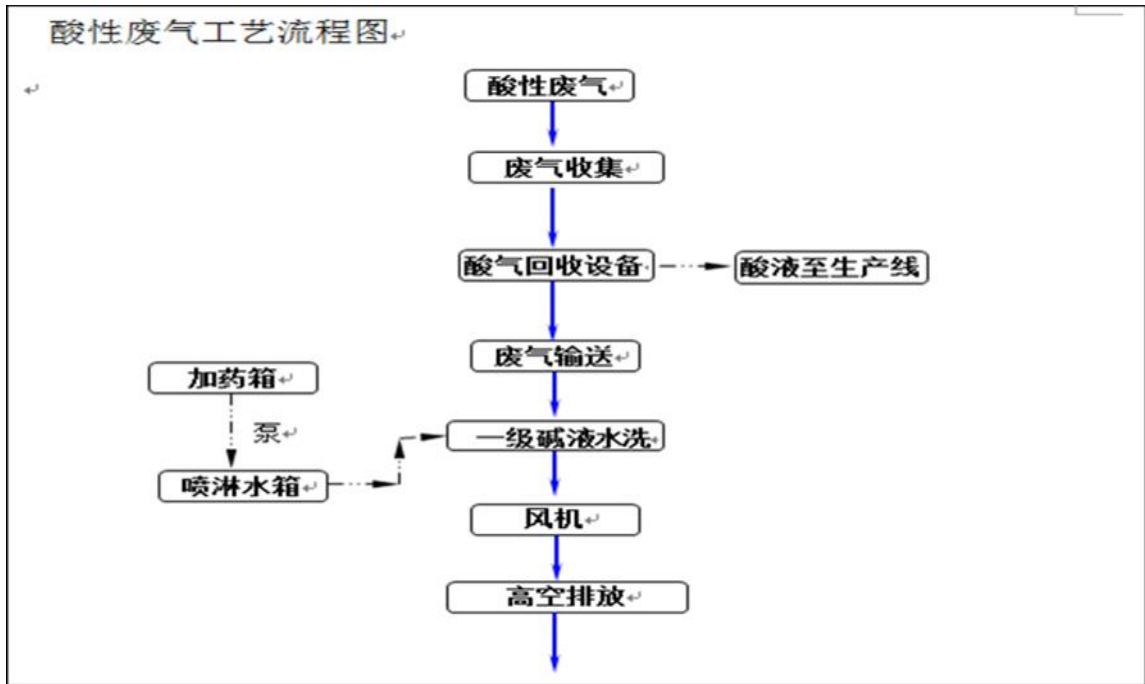
2 废气流处理工艺流程图
